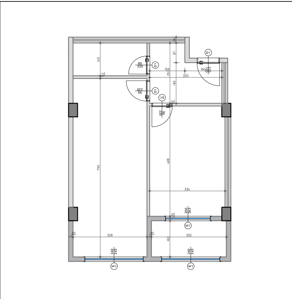
PLANIMETRIA E APARTAMENTIT - PERMASIM
